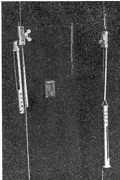
Fiskertermometer. Tilv. før nedfiring, tilh. under ophaling med slippeloddet sittende oppaa. I midten sees et termometer uttat av vendemekanismen.
