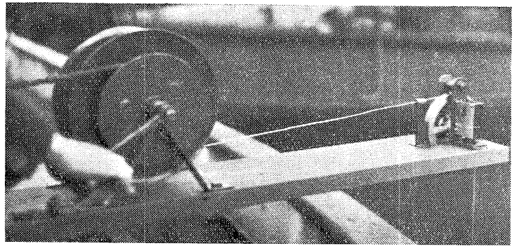
Loddemaskine til fiskeribruk. Til høire sees maaleskiven med dybdeviser, tilvenstre, over haanden, sees snorbremsen.
