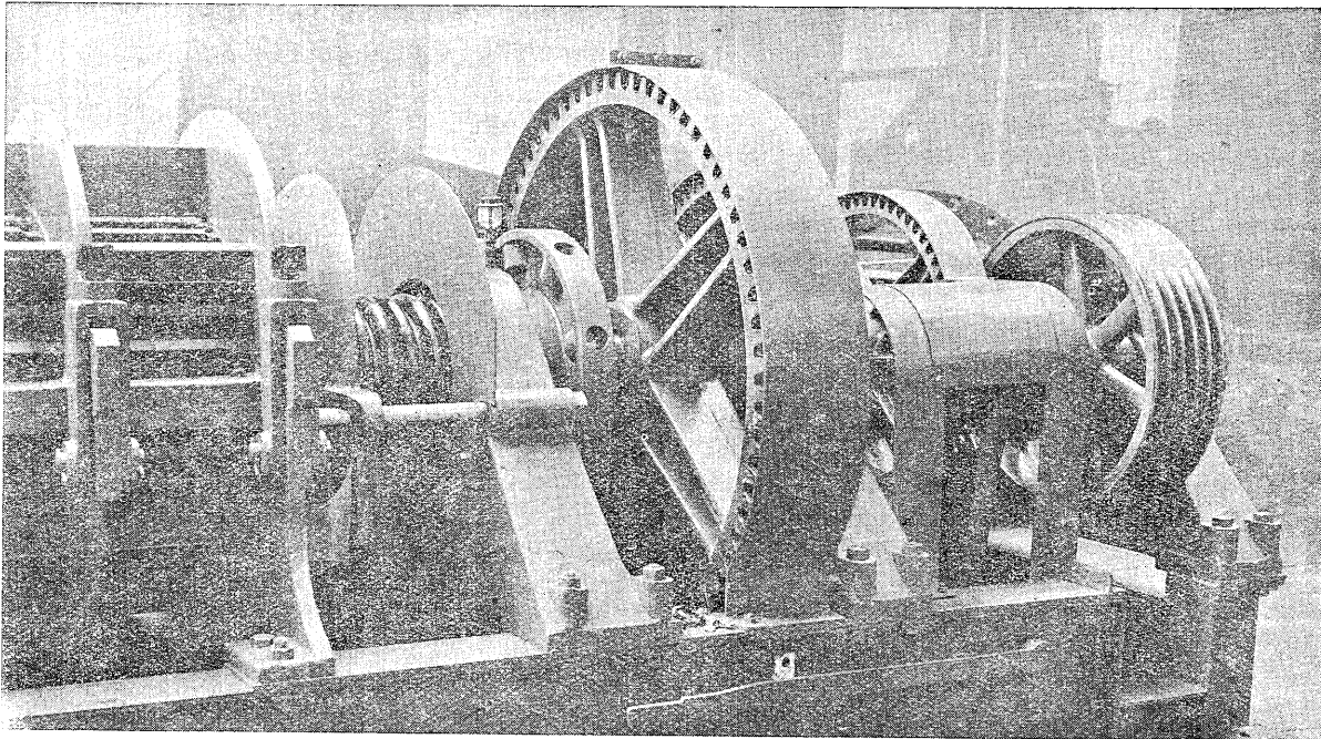
Driftanordningen for en Myren skrupresse. Legg merke til den kraftige konstruksjonen.
