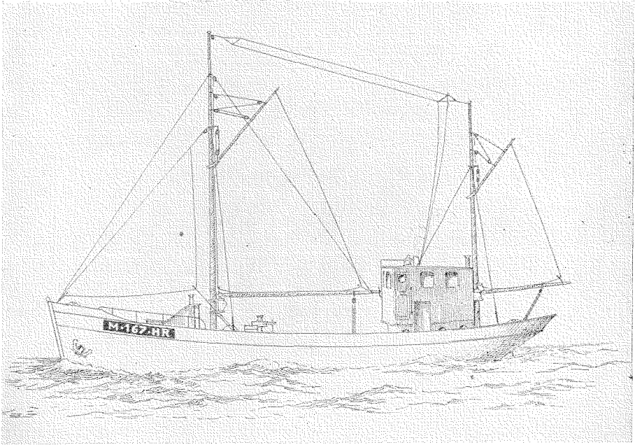
Fig. 5. Motorkutter med merke av 2. klasses størrelse.
