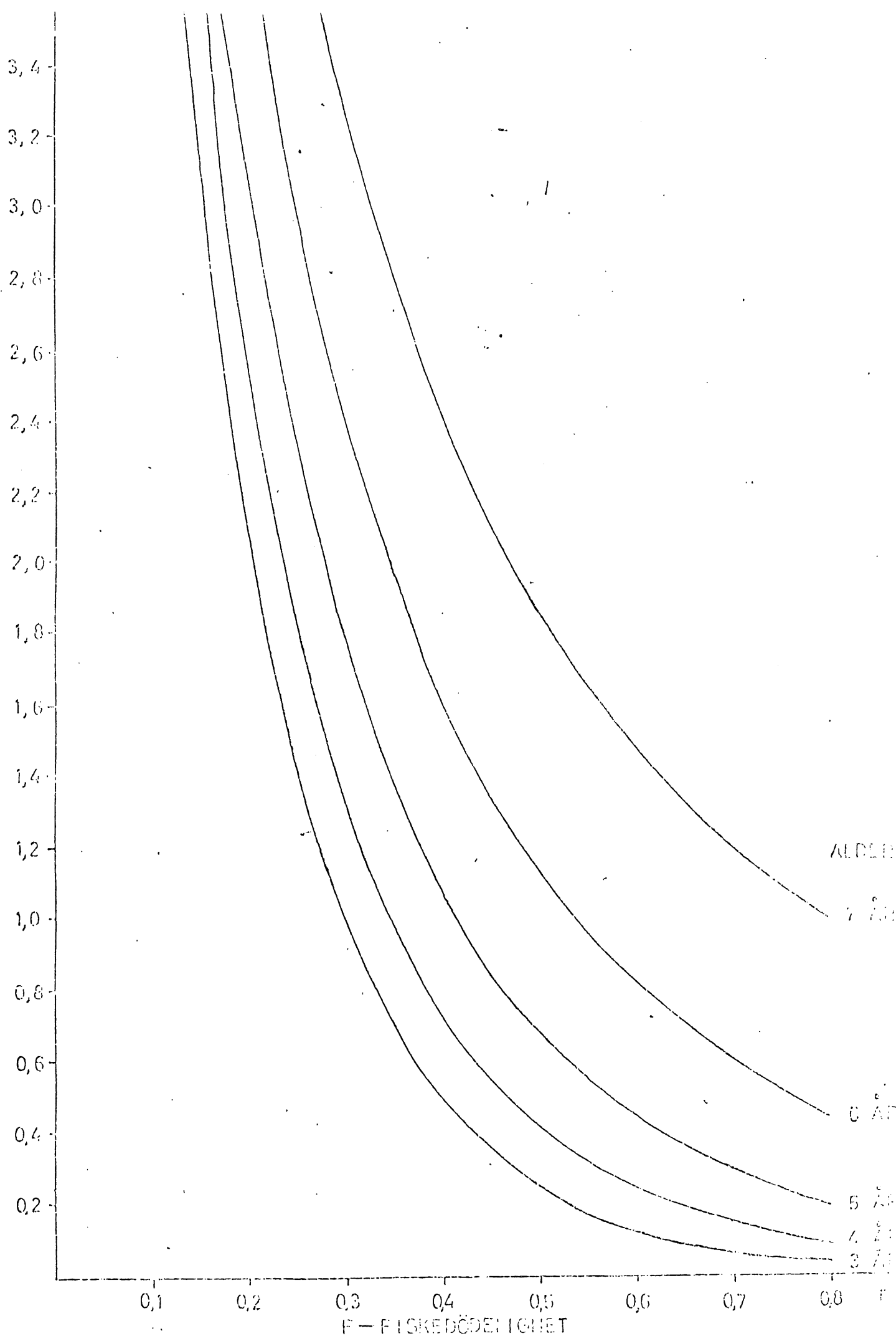
Fig. 2. Norsk arktisk torsk. Teoretisk sammenheng mellom fiskefølsomhet (fangeandelen) og avkastning i tonn ved en laveste bestandsnivå (beredningsnivå 7, 4, 5, 6 og 7 år). Naturlig dødelighet 0,20.
