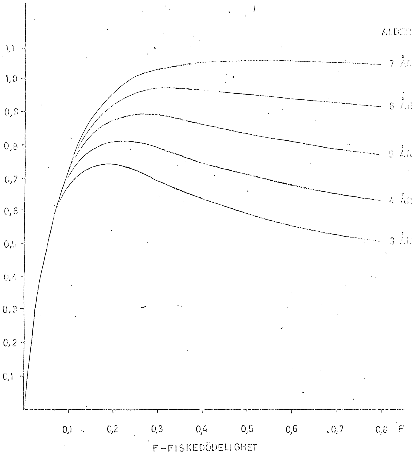
Fig. 1. Norsk arktisk torsk. Teoretisk sammenheng mellom fiskedødelighet (fangsttynnsats) og fangstutbytte i tonn ved en laveste beskætningsalder på henholdsvis 3, 4, 5, 6 og 7 år og gjennomsnittlig rekruttering. Naturlig dødelighet = 0,20.
