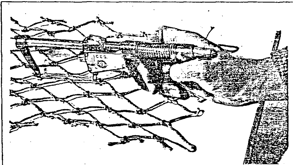
Figur 4.5: Illustrasjon av tre mulige posisjoner for måling av maskevidden. Spesielt viktig er det å plassere "pistol" eller målebrettet (trankanlbrettet) på en bestemt plass i maskene når den gjennomsnittelige maskevidden i en pose skal måles. Felikilden øker med økt trådtykkelse og størrelse av knutene (og dobbeltråd).
