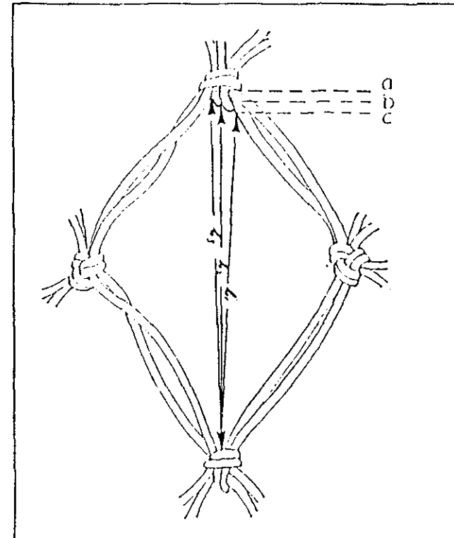
Figur 4.5: Illustrasjon av tre mulige posisjoner for måling av maskevidden. Spesielt viktig er det å plassere "pistol" eller målebrettet (trankanlbrettet) på en bestemt plass i maskene når den gjennomsnittelige maskevidden i en pose skal måles. Felikilden øker med økt trådtykkelse og størrelse av knutene (og dobbeltråd).
